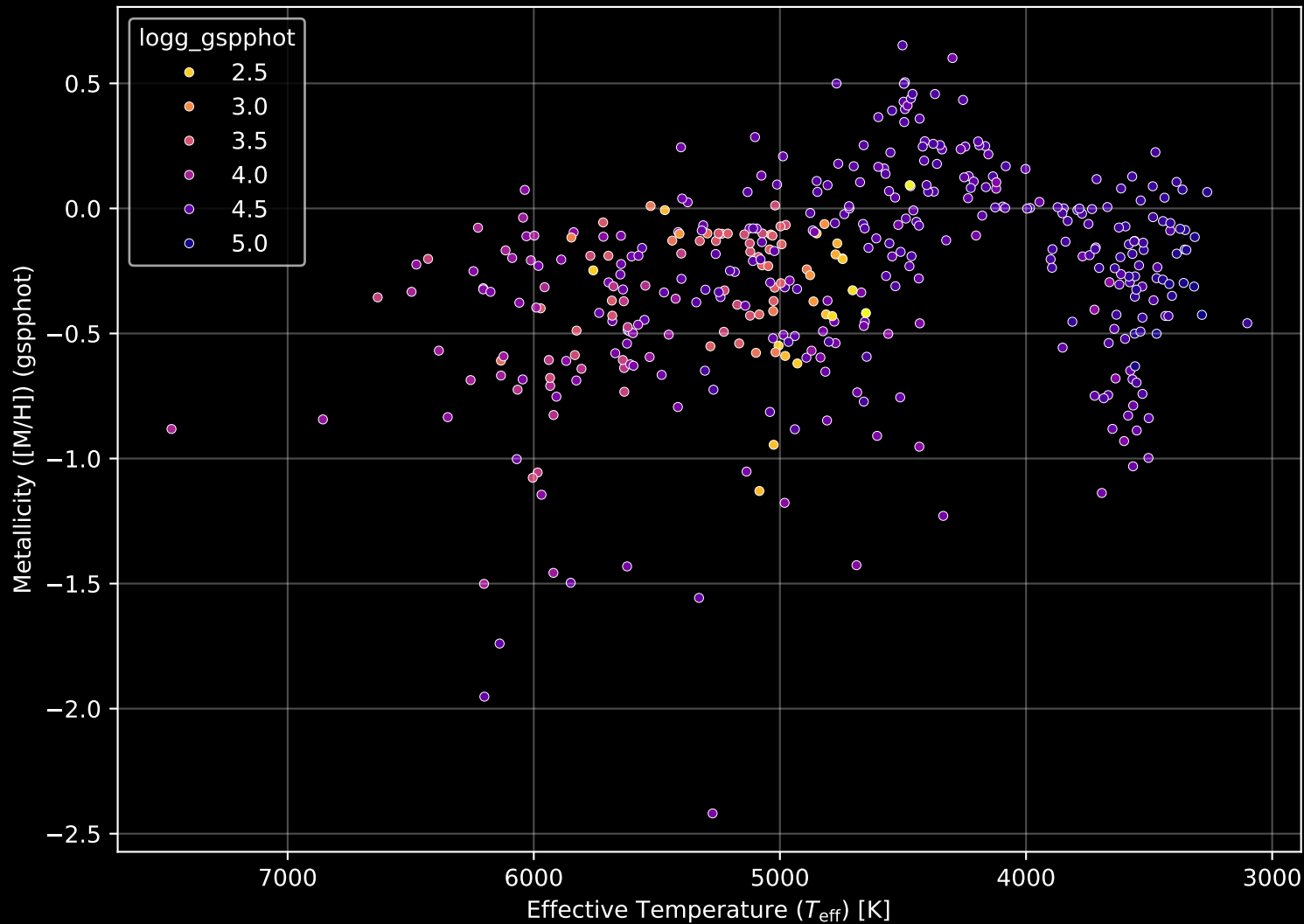
APOGEE DR17 Field: [060+75] Stellar Population Parameters (n= 406)
